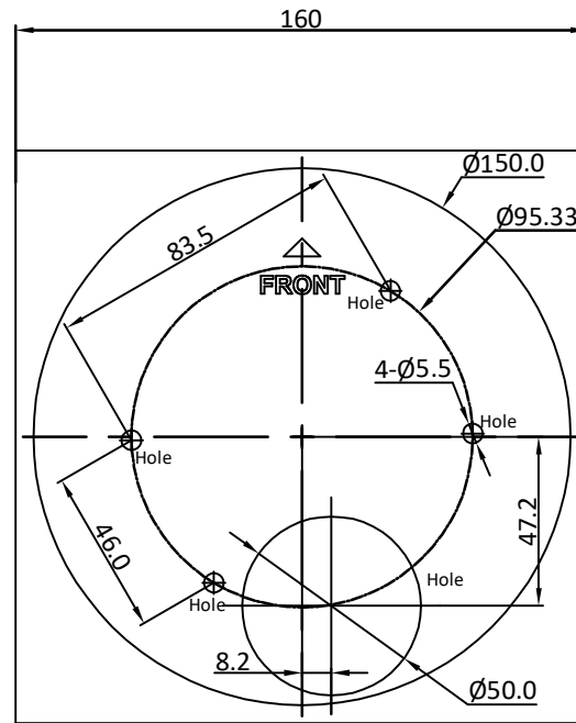
安装孔位
