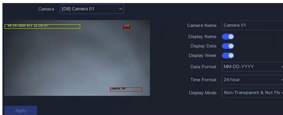
図 5-11 OSD
