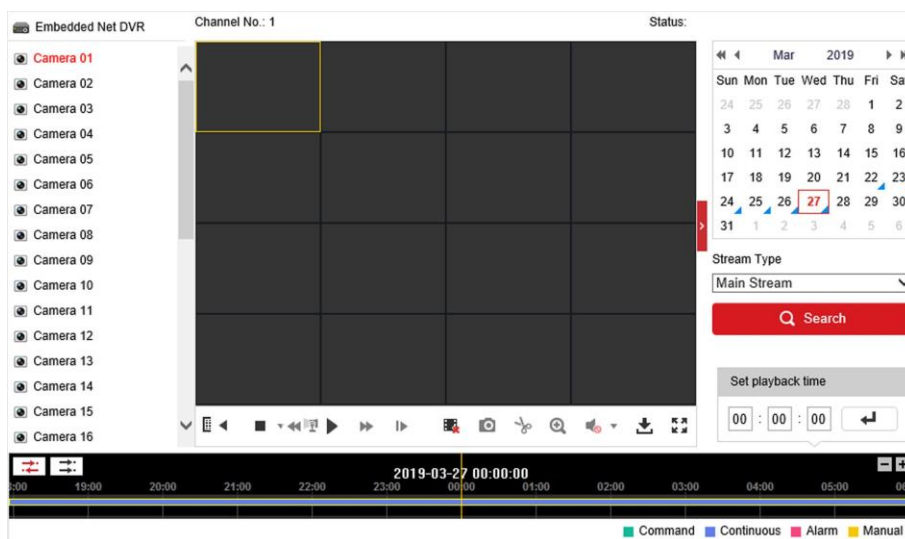
図 9-3 再生
