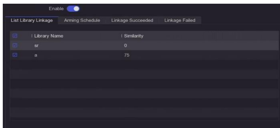
図 6-23 顔画像比較
