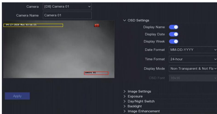
図 6-14 OSD
