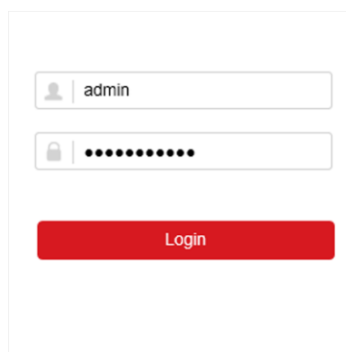
図 9-1 ログイン
