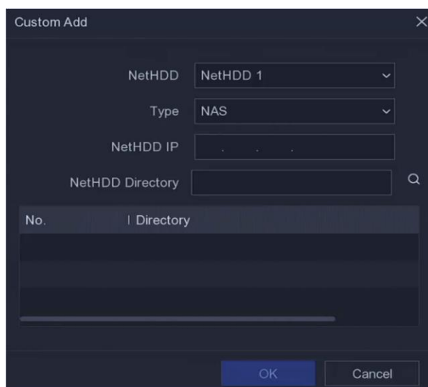
図 6-28 NetHDDの追加
