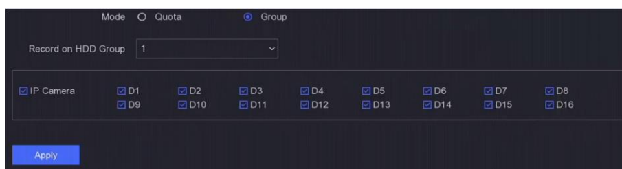
図 6-29 グループ
