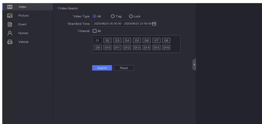
図 4-1 検索
