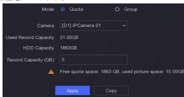
図 6-30 割り当て
