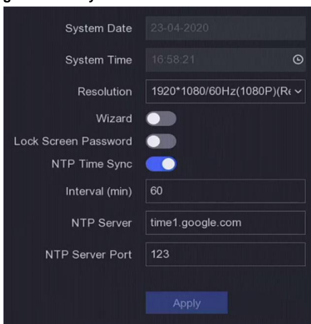
図 5-1 全般設定
