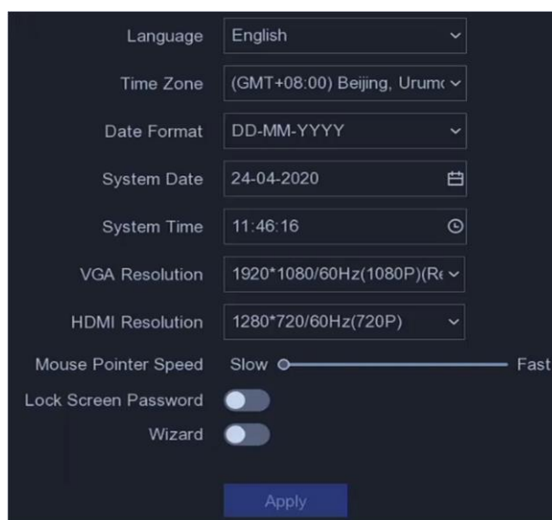
図 6-1 基本設定
