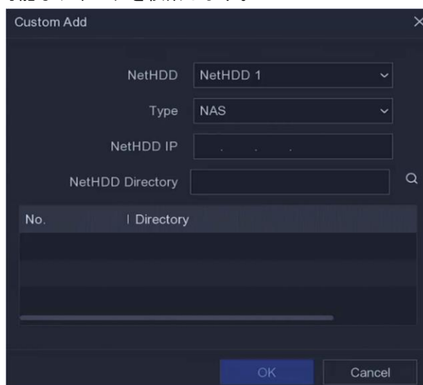
図 5-13 NetHDDの追加
