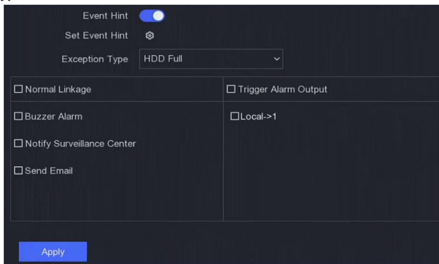
図 6-21 異常
