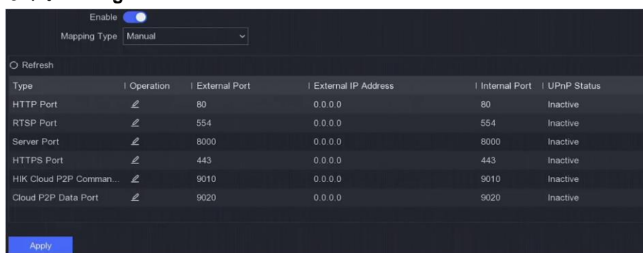
図 6-5 NAT
